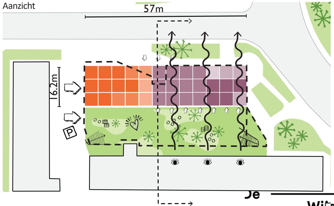
Plattegrond - daktuin niveau
